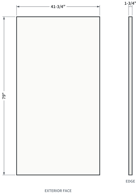
FIG. 1 ELEVATION AND EDGE VIEW
