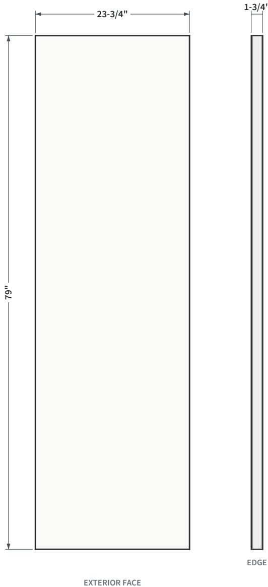
FIG. 1 ELEVATION AND EDGE VIEW
