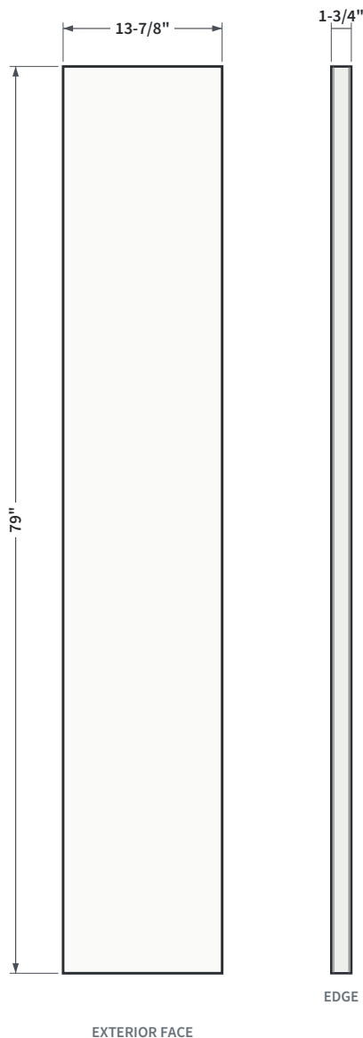
FIG. 1 ELEVATION AND EDGE VIEW
