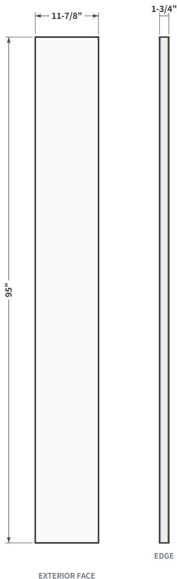
FIG. 1 ELEVATION AND EDGE VIEW
