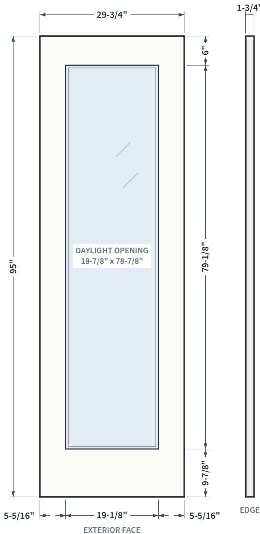
FIG. 1 ELEVATION AND EDGE VIEW
