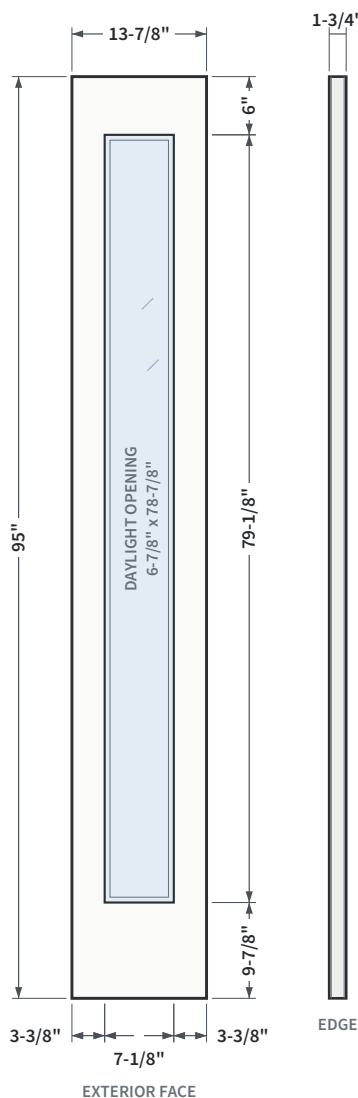
FIG. 1 ELEVATION AND EDGE VIEW
