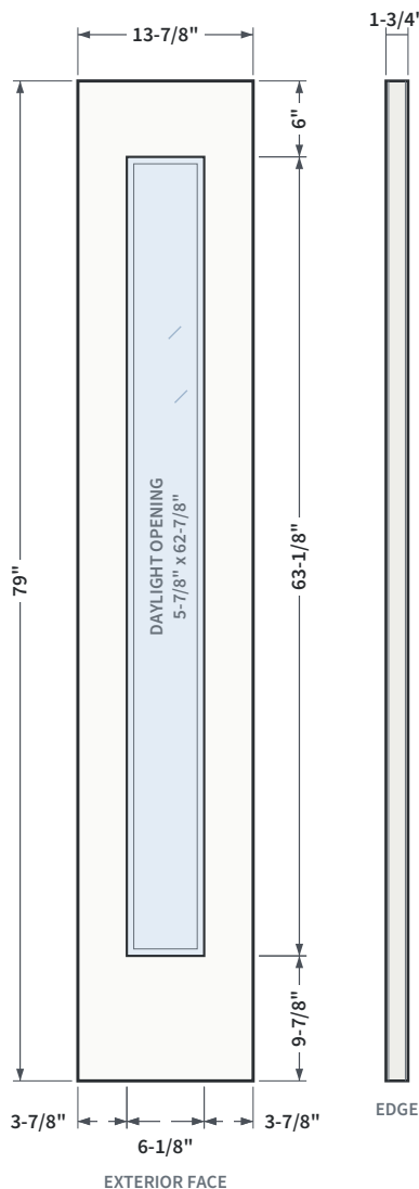
FIG. 1 ELEVATION AND EDGE VIEW
