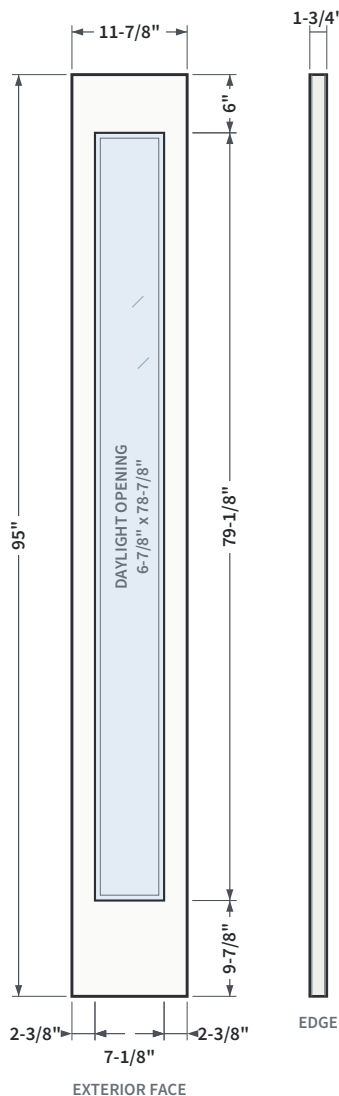
FIG. 1 ELEVATION AND EDGE VIEW
