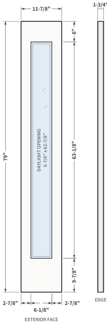
FIG. 1 ELEVATION AND EDGE VIEW
