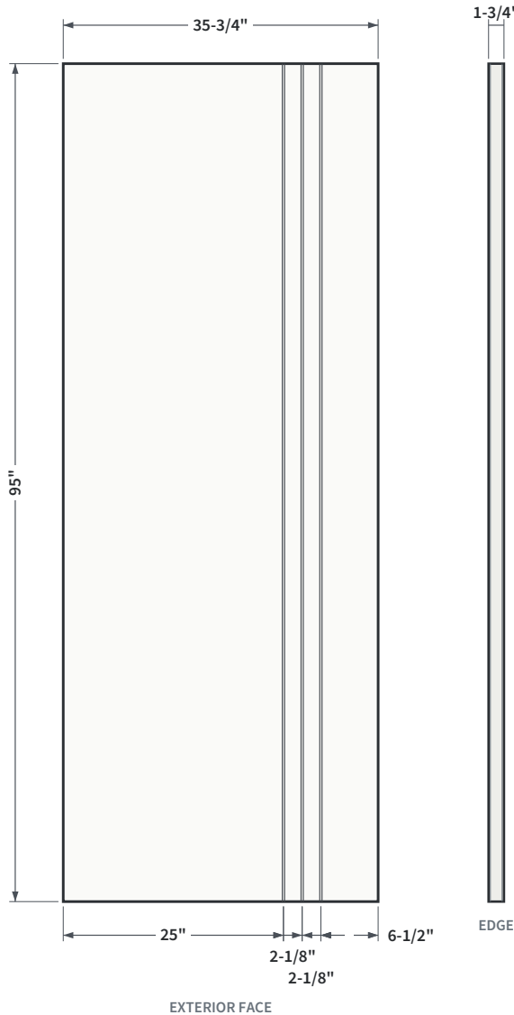
FIG. 1 ELEVATION AND EDGE VIEW
