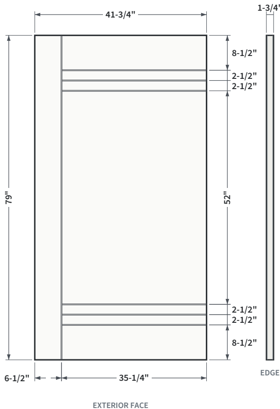
FIG. 1 ELEVATION AND EDGE VIEW
