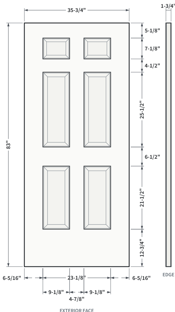
FIG. 1 ELEVATION AND EDGE VIEW
