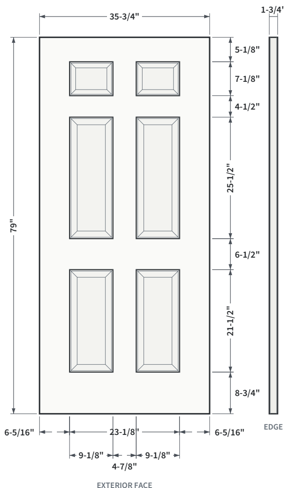
FIG. 1 ELEVATION AND EDGE VIEW
