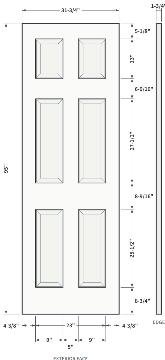
FIG. 1 ELEVATION AND EDGE VIEW
