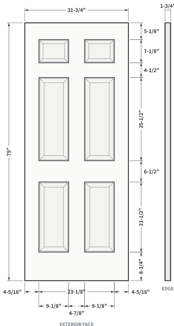
FIG. 1 ELEVATION AND EDGE VIEW
