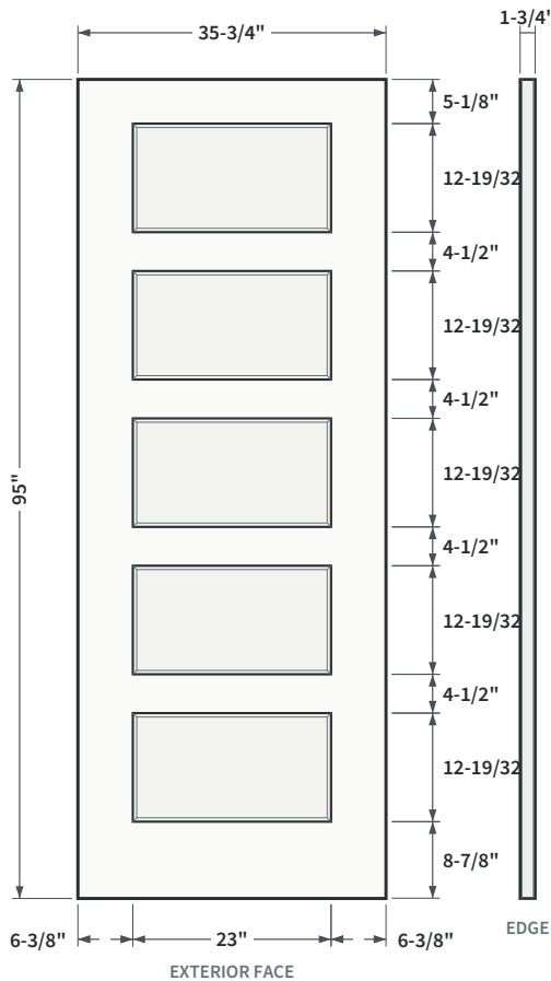
FIG. 2 SHAKER EMBOSSEMENT PROFILE
