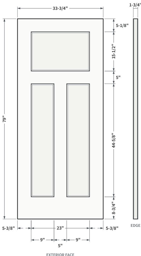
FIG. 1 ELEVATION AND EDGE VIEW
