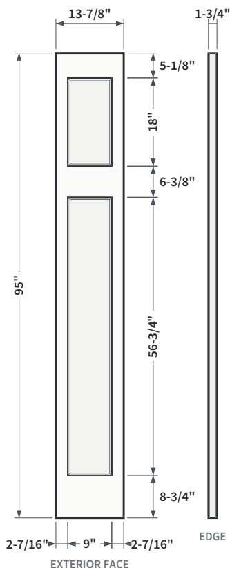
FIG. 2 SHAKER EMBOSSEMENT PROFILE
