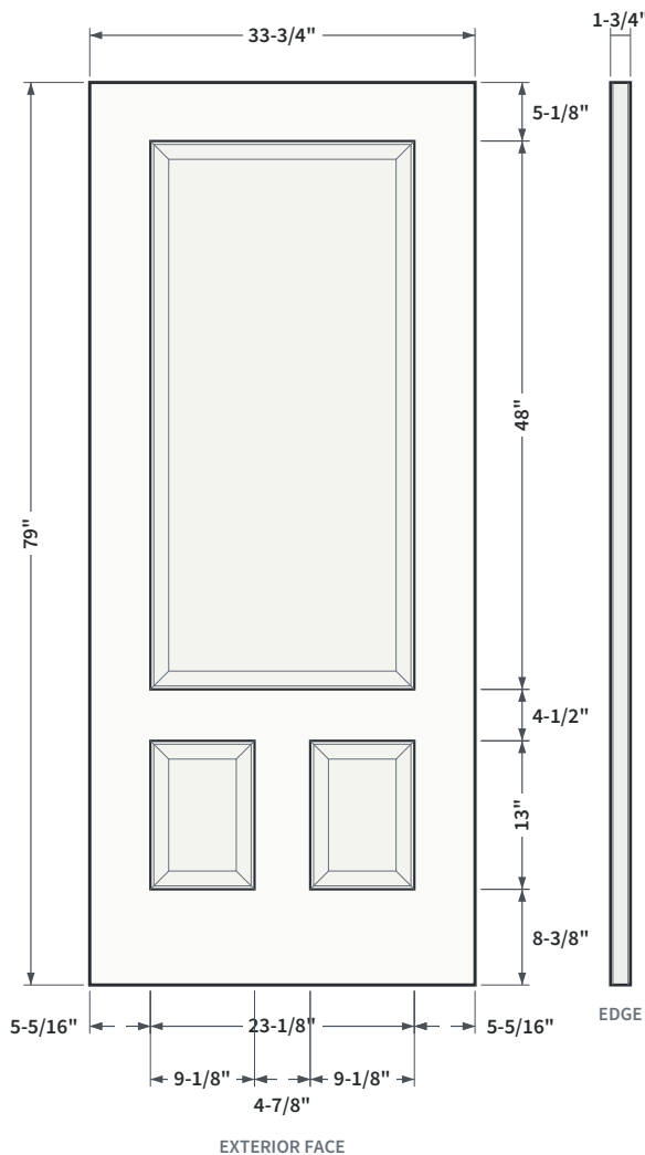
FIG. 1 ELEVATION AND EDGE VIEW
