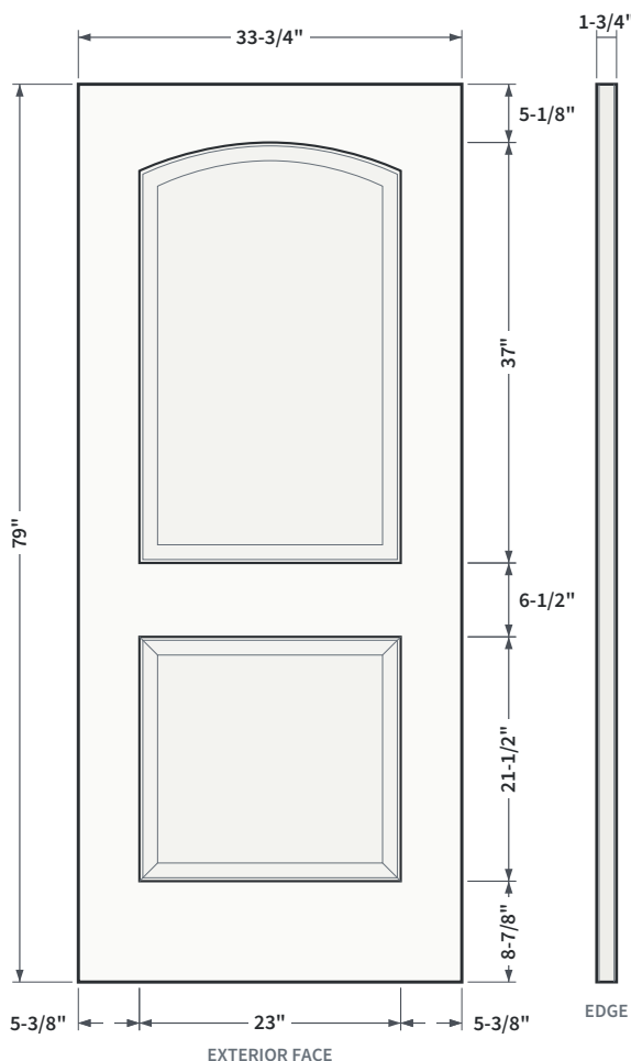
FIG. 1 ELEVATION AND EDGE VIEW
