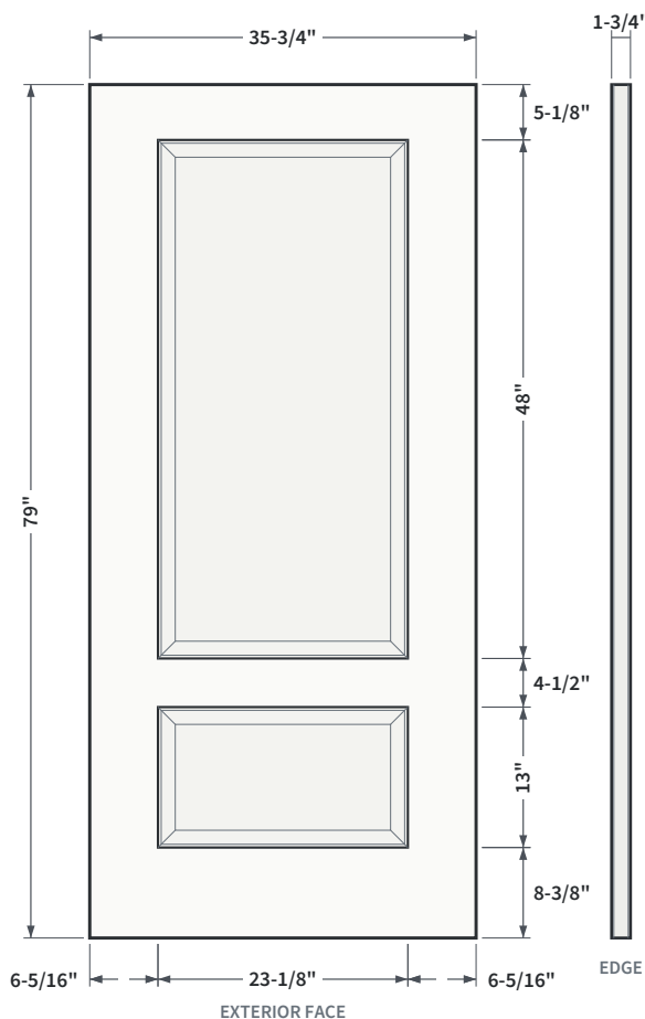
FIG. 1 ELEVATION AND EDGE VIEW
