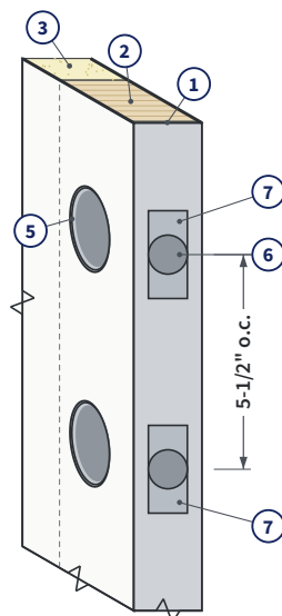
FIG. 4 LOCK EDGE DETAIL
