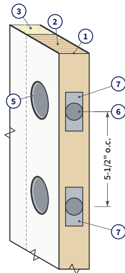
FIG. 3 LOCK EDGE DETAIL
